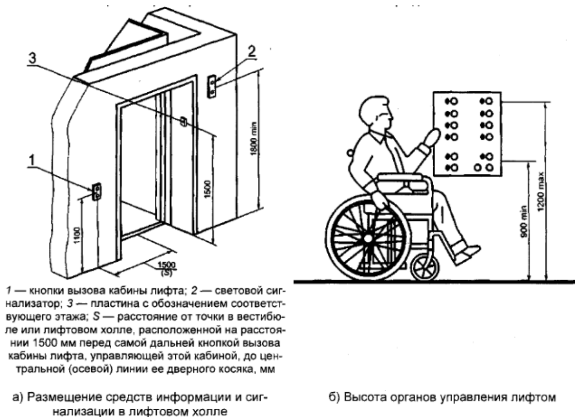
Рисунок 1 - Средства информации и сигнализации в лифтах
