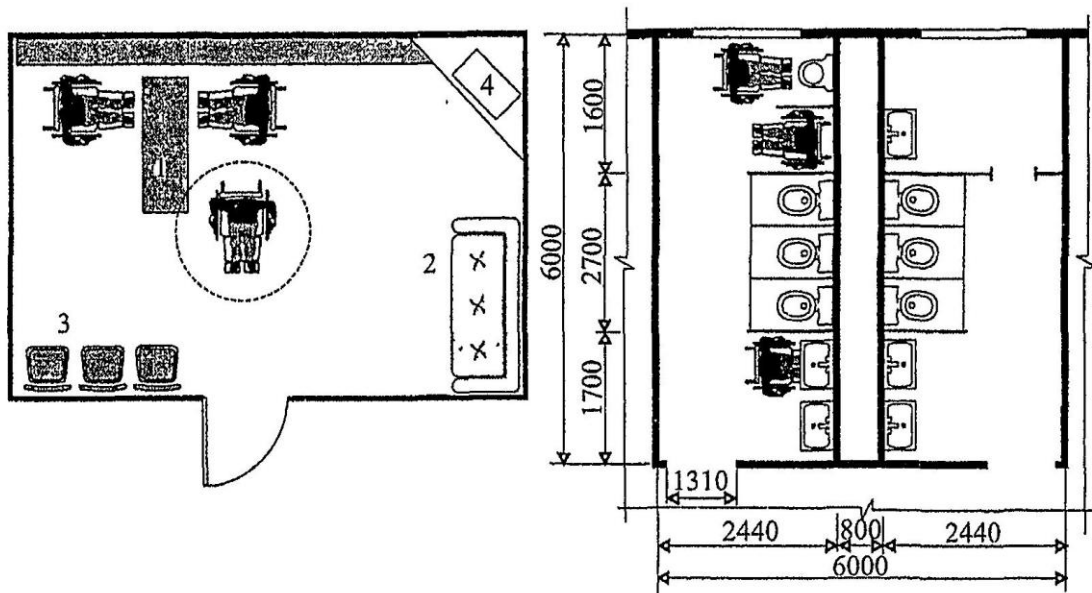
Встроенное помещение инвентарного типа для пассивного отдыха; пример оборудования комнаты отдыха для инвалидов: 1 – стол для настольных игр; 2 – диван; 3 – кресла; 4 – телевизор
