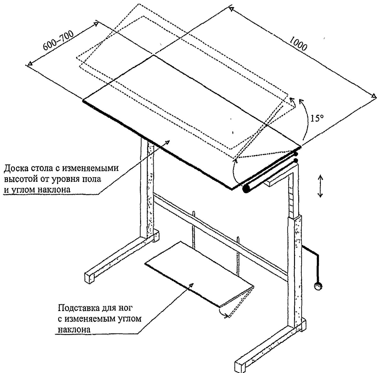
Рисунок В.12 – Трансформируемый рабочий стол для инвалида
