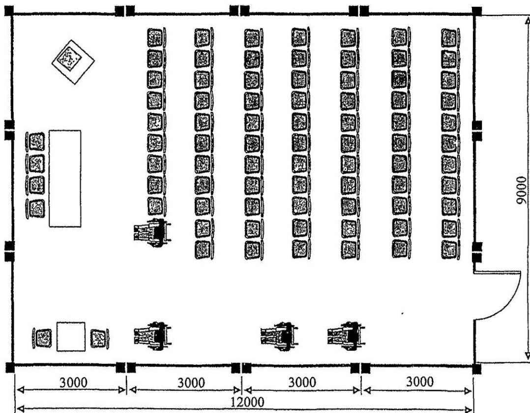
Места инвалидных колясок в помещении для собраний
