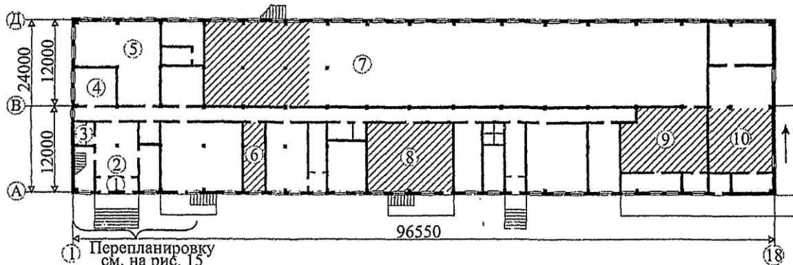
План на отм. 4800
