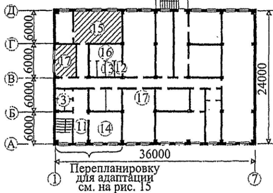
План на отм. 4800
